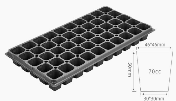
LXS50 L54*W28*H5cm
