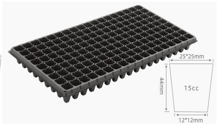
LXQA162 L54*W28*H4.4cm
