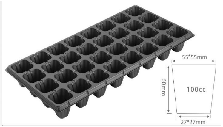
LXQA32 L54*W28*H6cm
