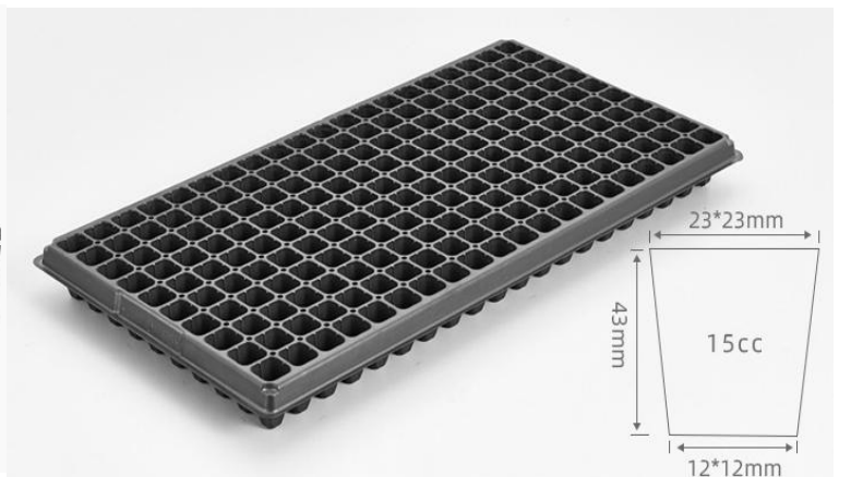
LXS200 L54*W28*H4.3cm
