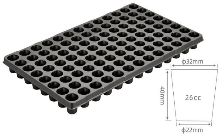
LXD104 L52.3*W30*H4cm
